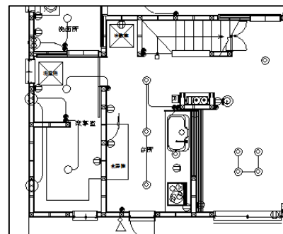
CAD 図面
